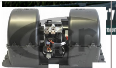
מאן (MAN) TGA / TGS - מנוע מפוח מושלם כולל נגד
