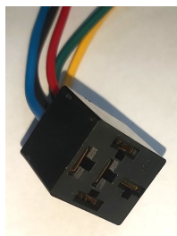
שקע לריליי 5 יציאות + חוטים SKU: FY-68B
