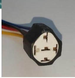
שקע לריליי 5 יציאות + חוטים קרמי
